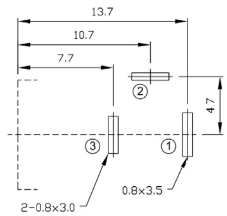
P.C.B LAYOUT(±0.1) (BOTTOM VIEW)
