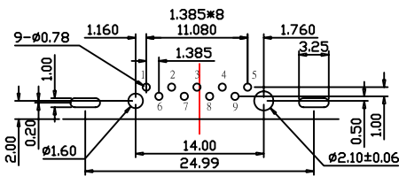
P.C.Board Layout
