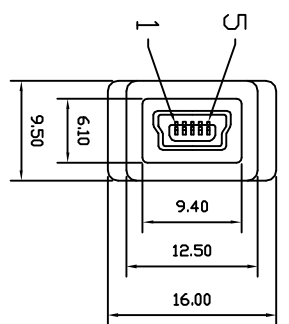
MINI USB 5P FEMALE
