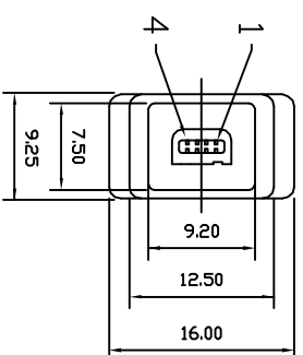
MINI USB 4P MALE
