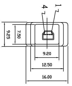
MINI USB 4P MALE MISTUMI
